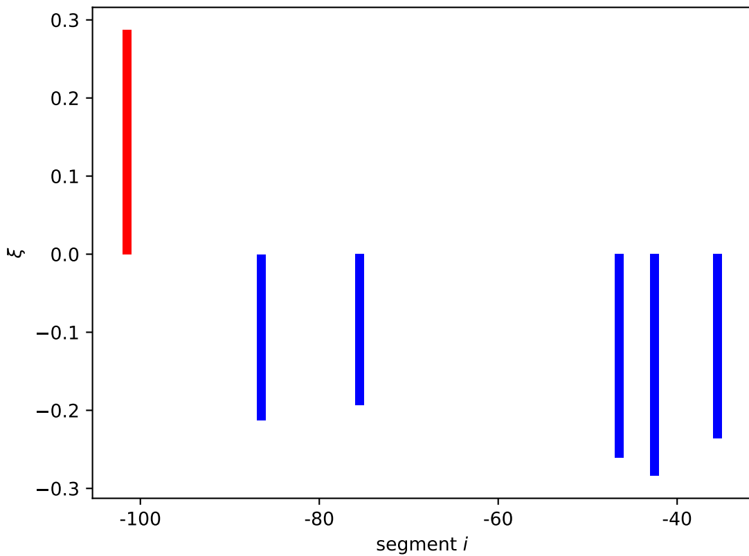
xylF expression shift \xi_i[11]
