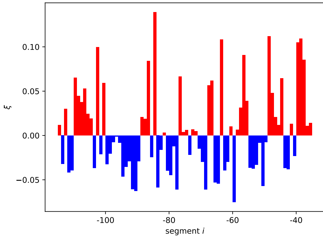
xylF expression shift \xi_i[11]
