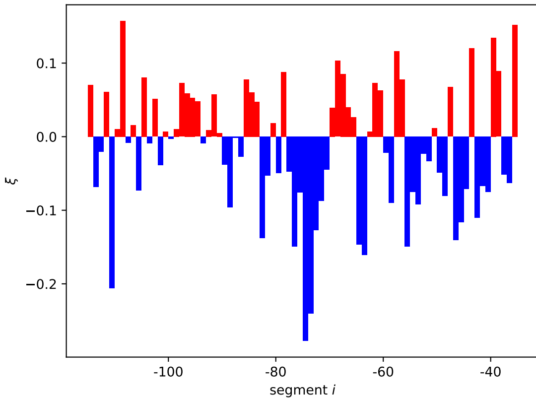
ybeZ expression shift \xi_i[11]
