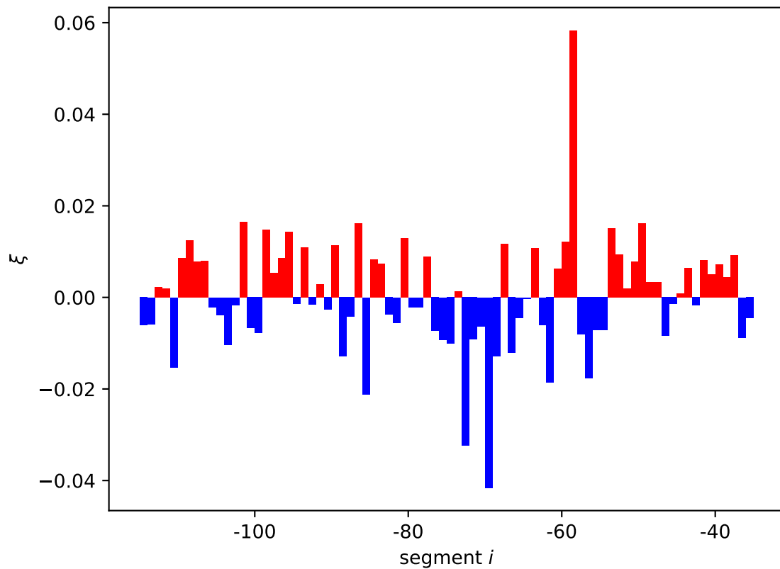
yecE expression shift \xi_i[01, 10]
