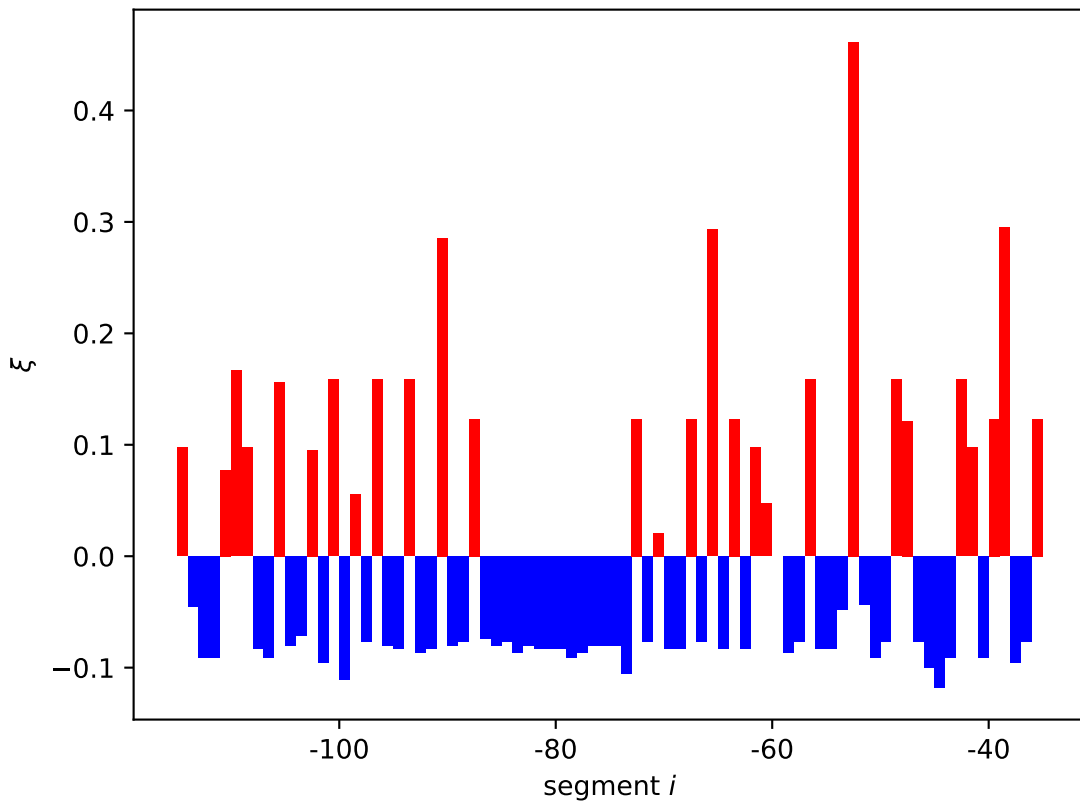
yecE expression shift \xi_i[01, 10]
