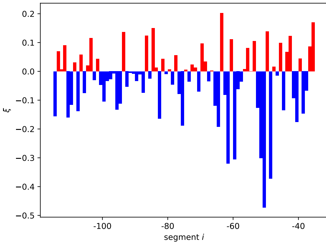
yedK expression shift \xi_i[11]
