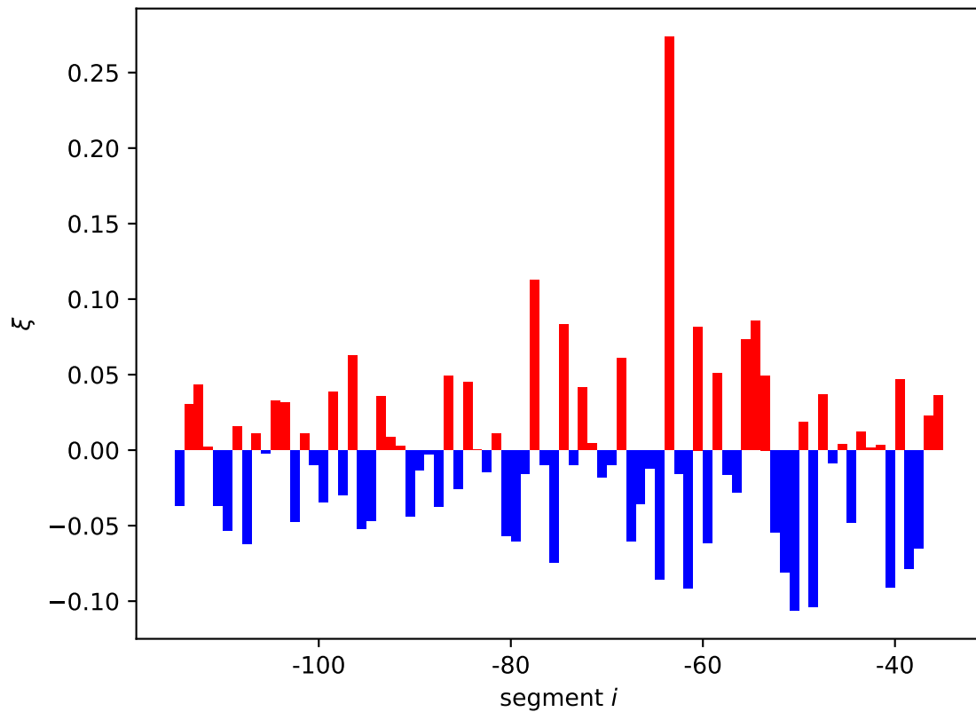
yedK expression shift \xi_i[11]
