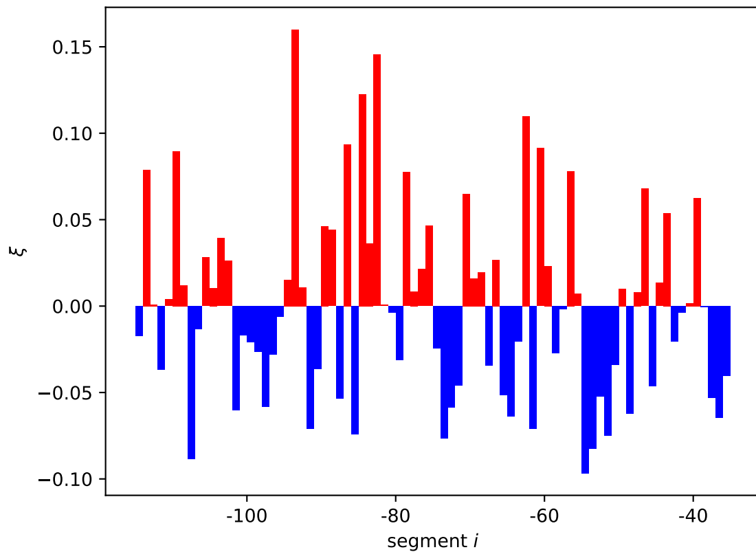
yehS expression shift \xi_i[11]
