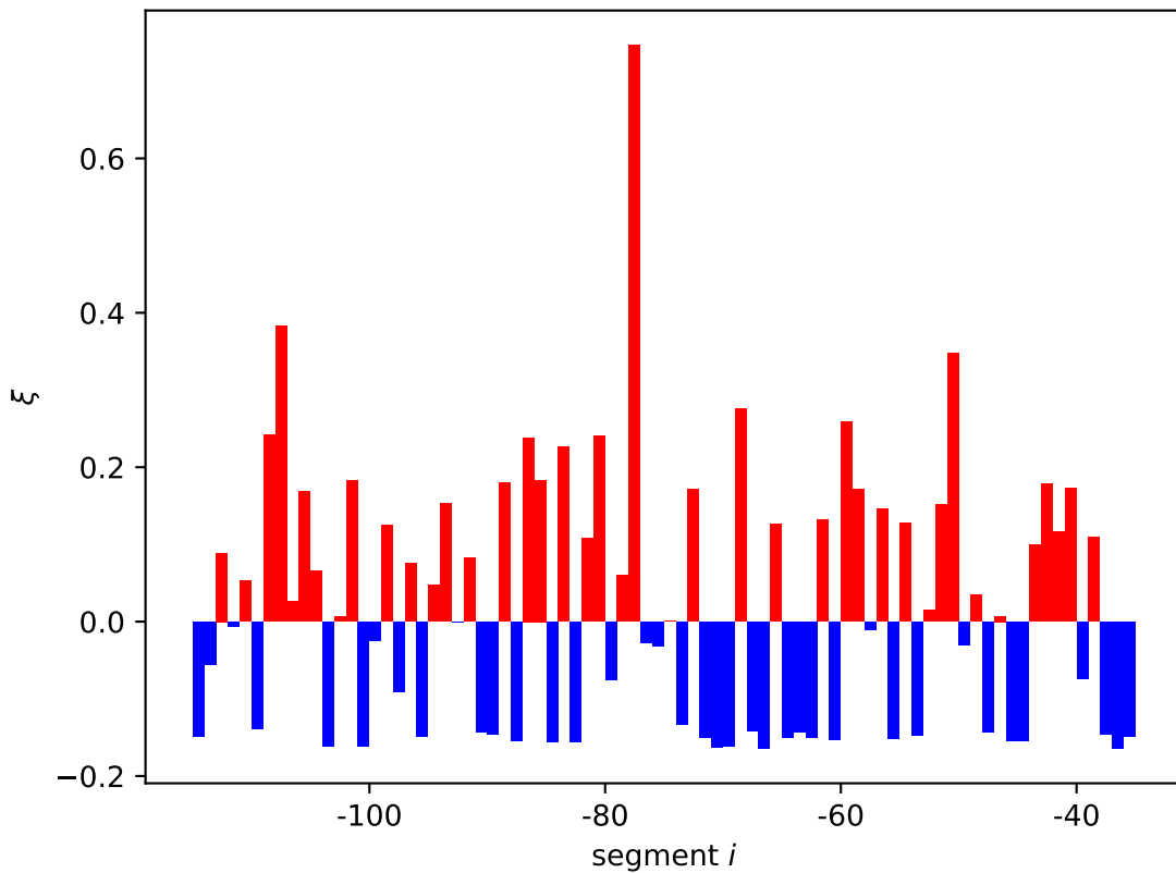
yehT expression shift \xi_i[11]
