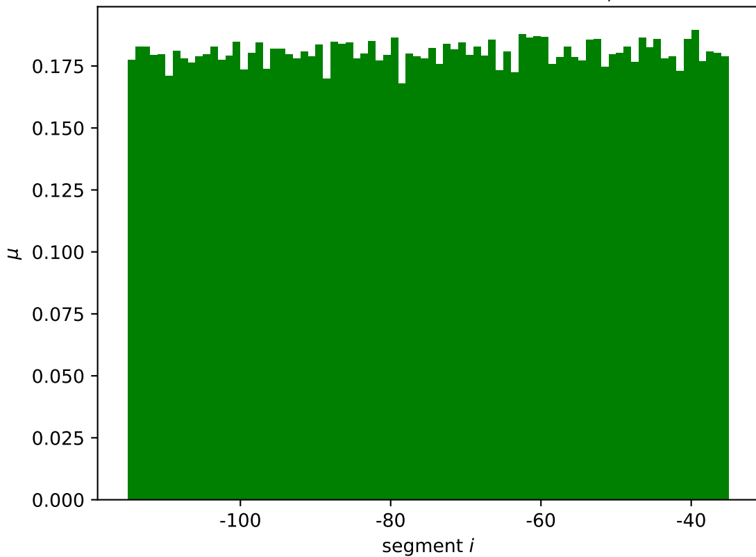
yehT mean wildtype expression \mu_i^*
