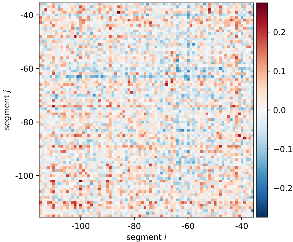
yehT expression shift \xi_{i,j}[0101, 0110, 1010]
