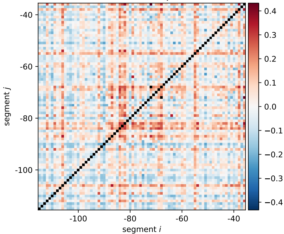
yehT expression shift \xi_{i,j}[0011, 1100]
