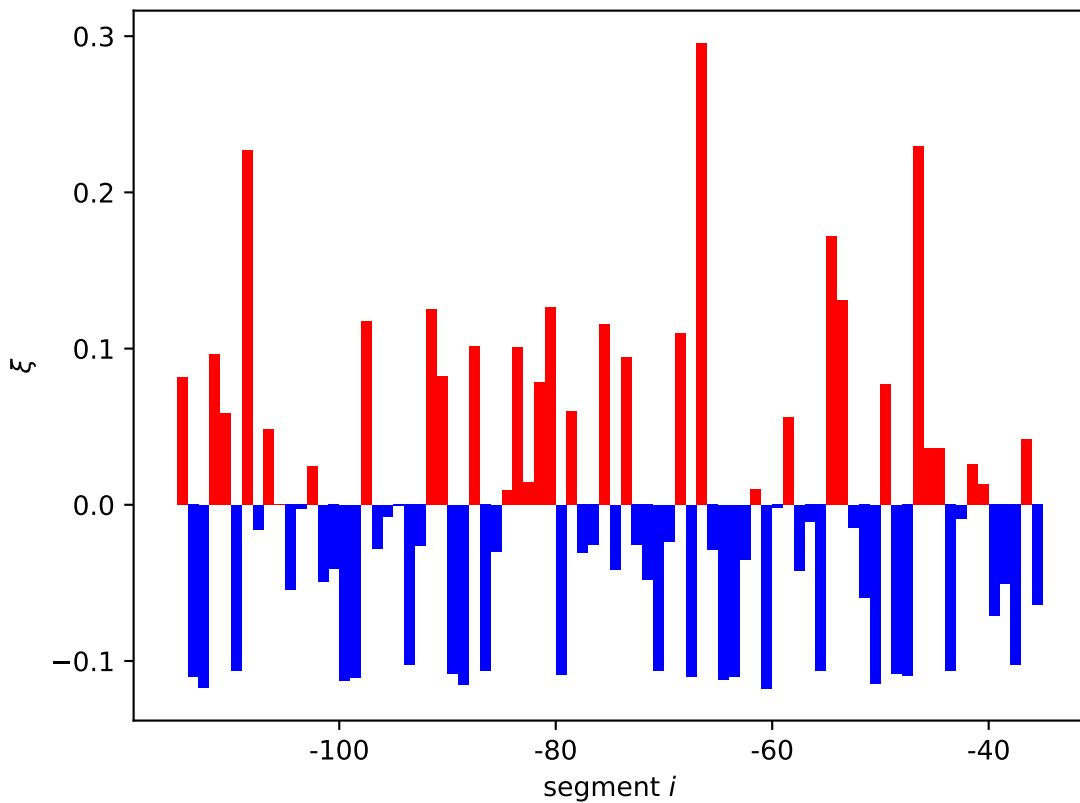
yfhG expression shift \xi_i[11]
