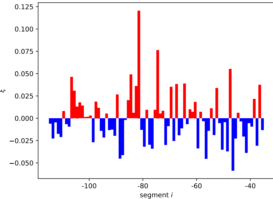
yfhG expression shift \xi_i[11]
