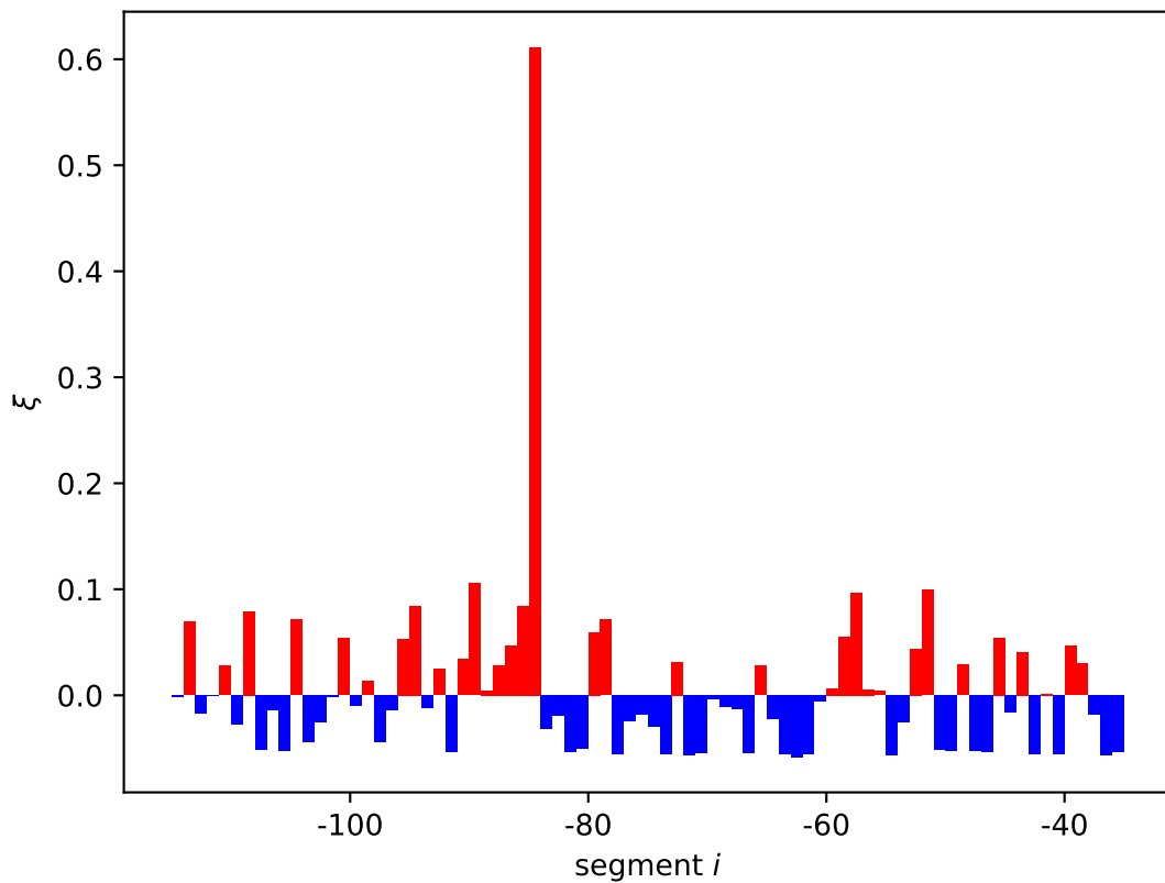
ygeR expression shift \xi_i[11]
