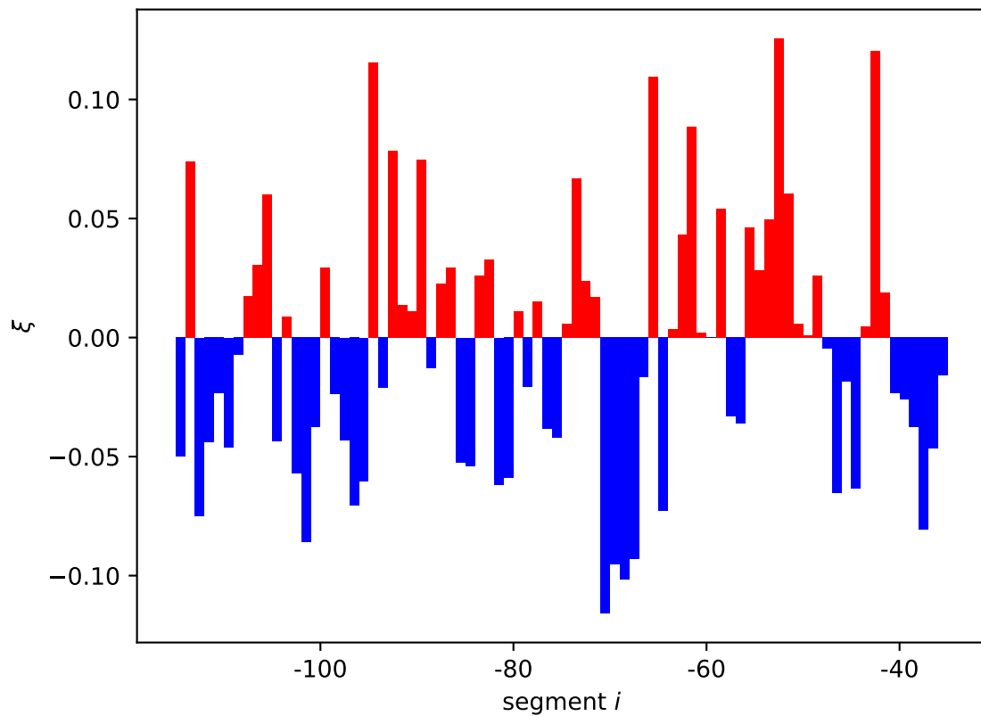
ygjP expression shift \xi_i[11]
