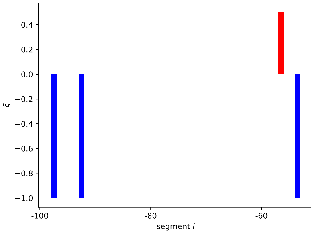
ymgG expression shift \xi_i[11]
