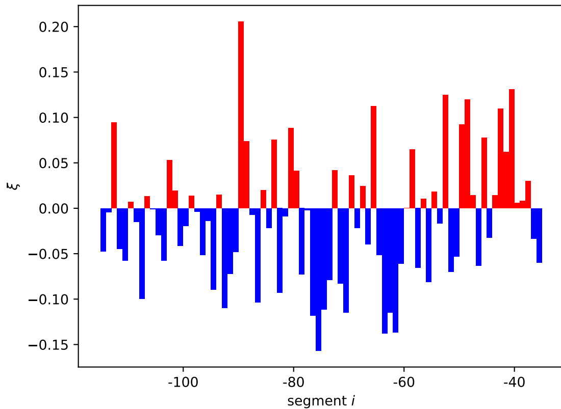
zapB expression shift \xi_i[11]
