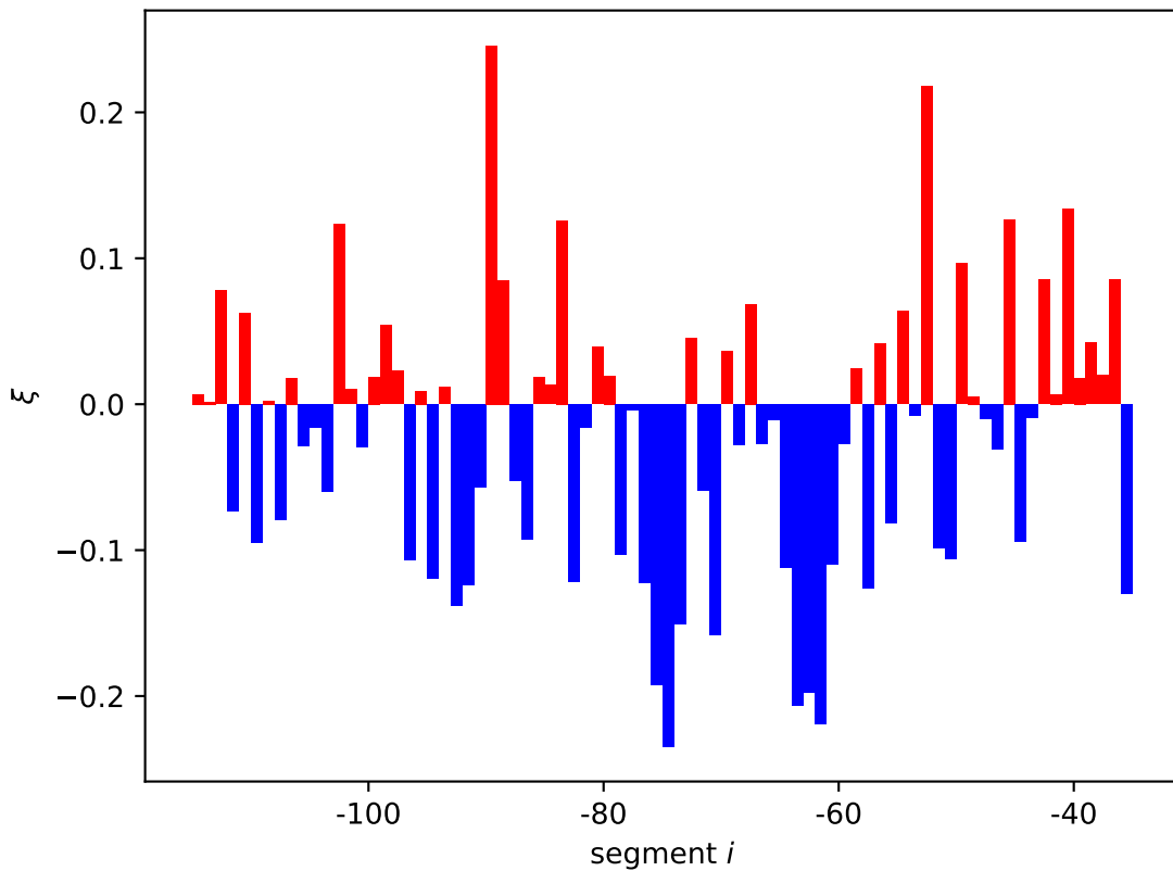
zapB expression shift \xi_i[11]
