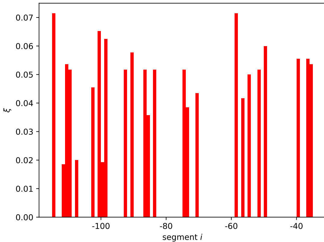
znuCB expression shift \xi_i[11]
