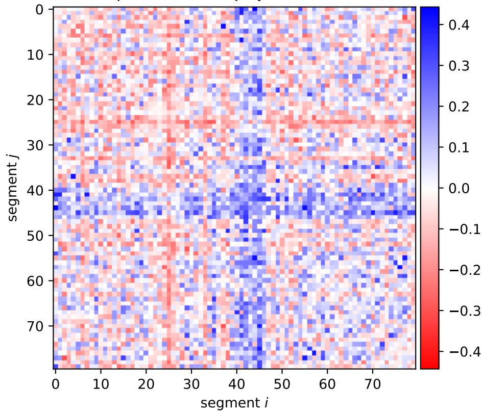
Expression shift \xi[i, j; (0, 1), (0, 1)]
