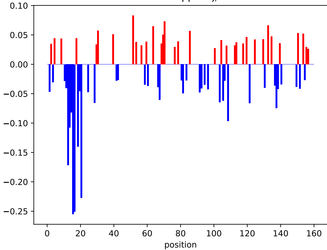
Boostrapped \xi_i
