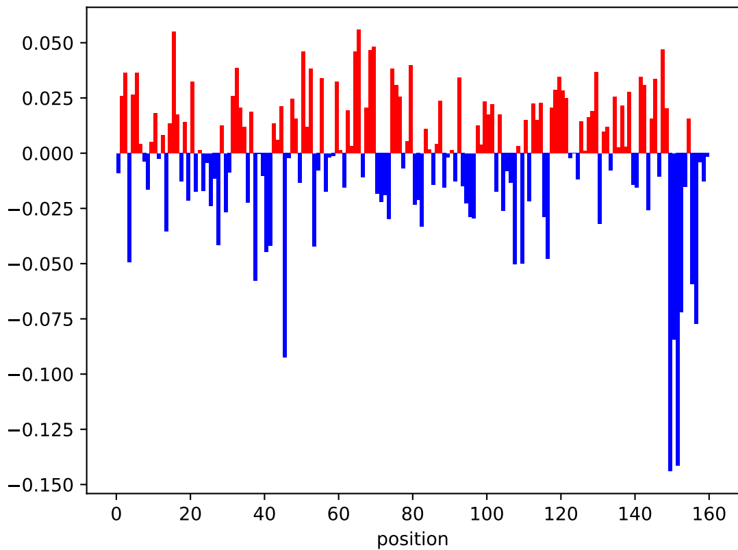
Boostrapped \xi_i
