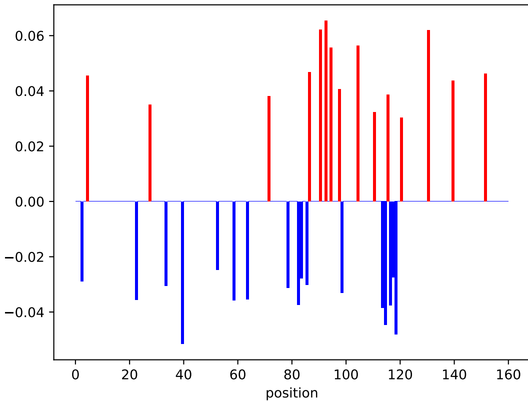
Boostrapped \xi_i
