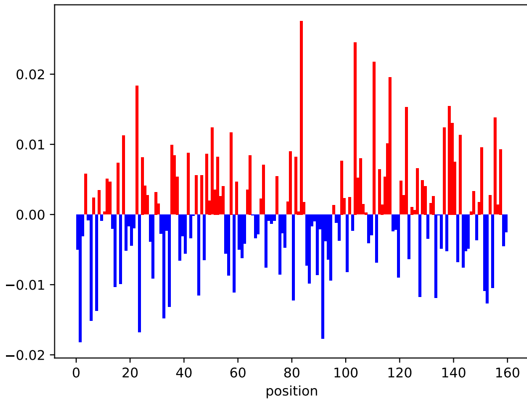
Boostrapped \xi_i
