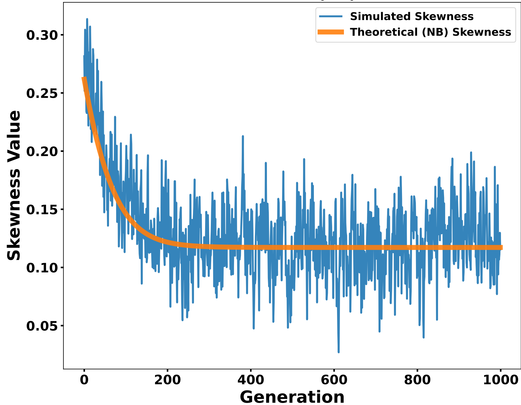
Skewness (NB)
