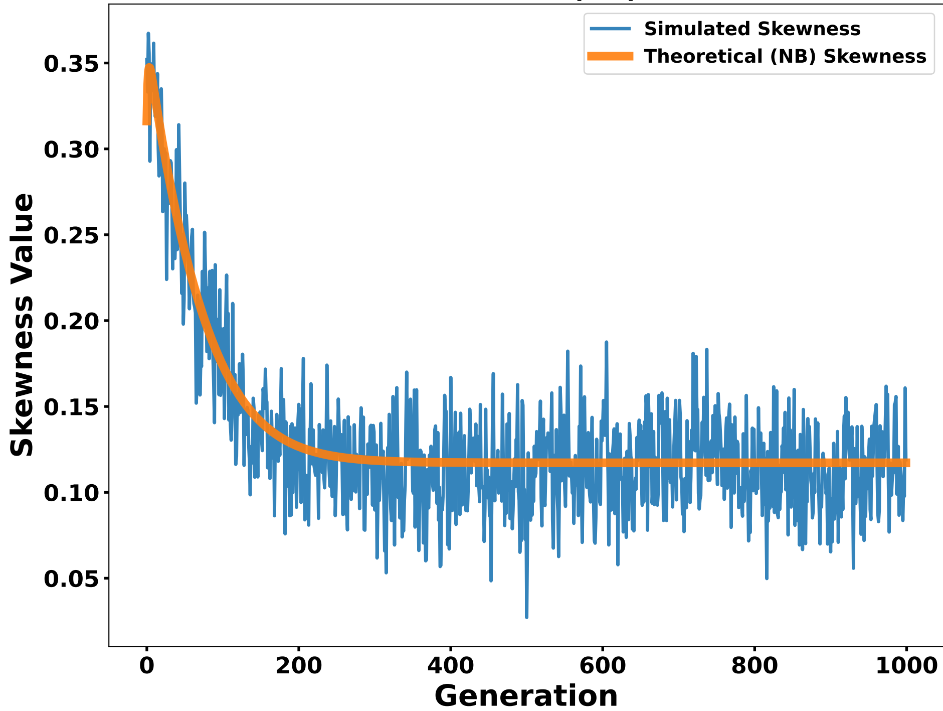
Skewness (NB)
