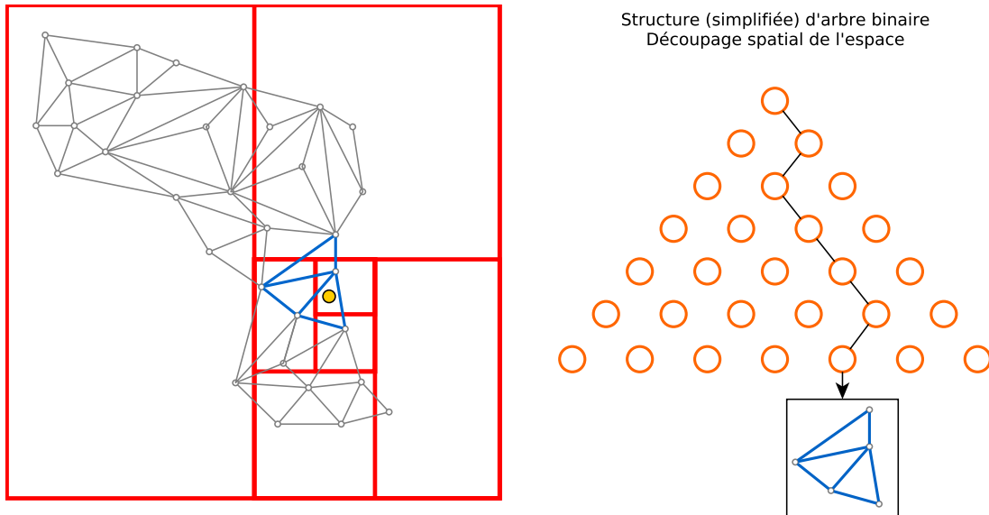
FIGURE 3 – Recherche optimisée d'éléments d'un maillage via une structure d'arbre binaire. La feuille de l'arbre contenant le point jaune est trouvée en 6 évaluations (arcs noirs dans la structure d'arbre). Cette feuille contient un nombre réduit de triangles (ici, 3), ce qui limite significativement le nombre d'opérations coûteuses ainsi que la complexité générale de l'algorithme. Les recherches basées sur des arbres binaires sont généralement de complexité en \mathcal{O}(\log(n)) .
