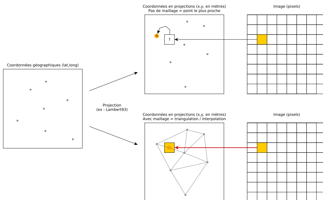
FIGURE 2 – Passage de coordonnées géographiques aux pixels d'une image. La fonction recherchant un point projeté à partir des coordonnées d'un pixel de l'image peut être longue à l'exécution. Il devient nécessaire de réfléchir à une optimisation permettant d'éviter de parcourir tous les points projetés pour trouver le point correspondant à notre pixel (sans optimisation : complexité en \mathcal{O}(n) ).
