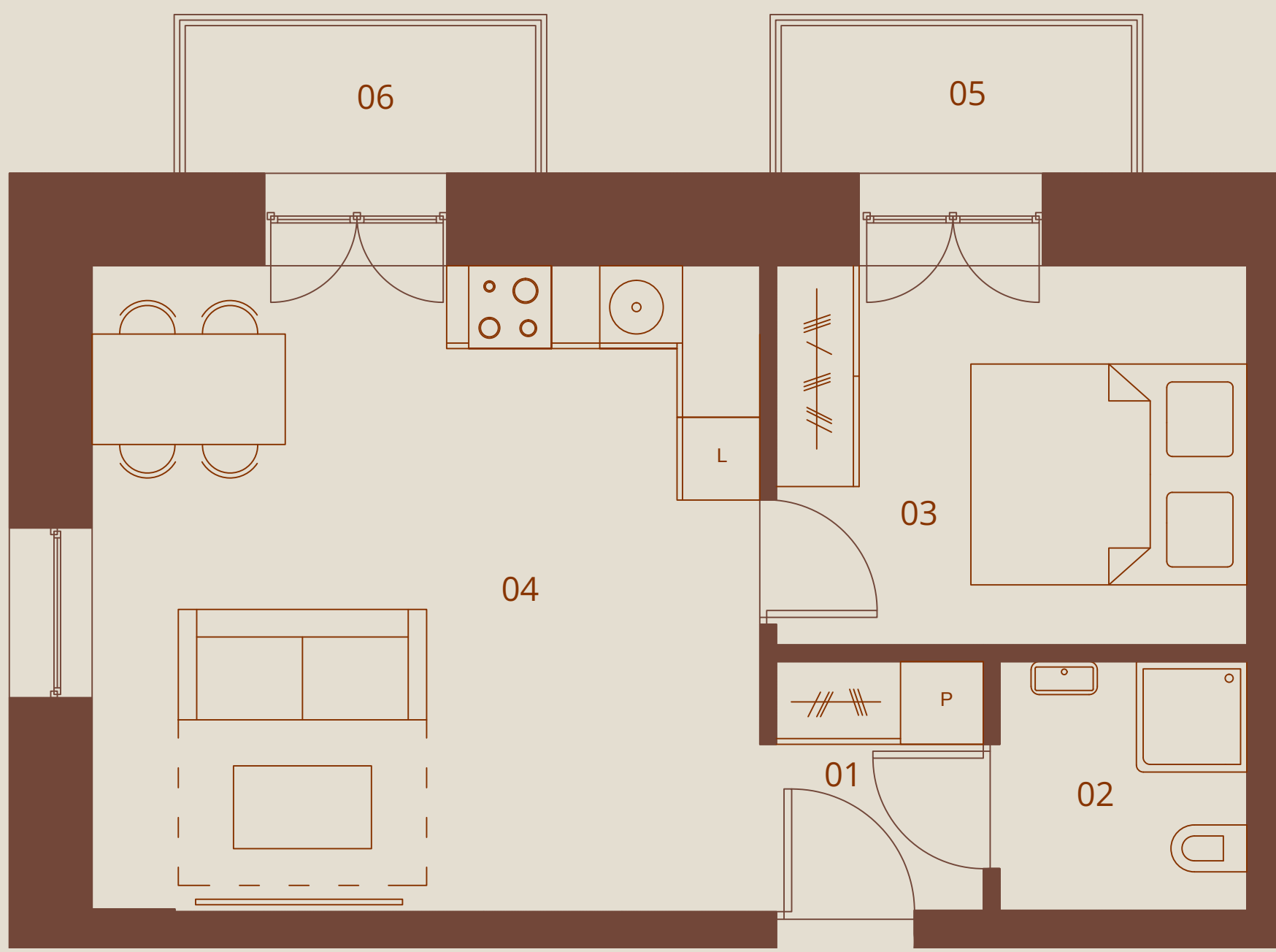
Plan piętra 1-ego
