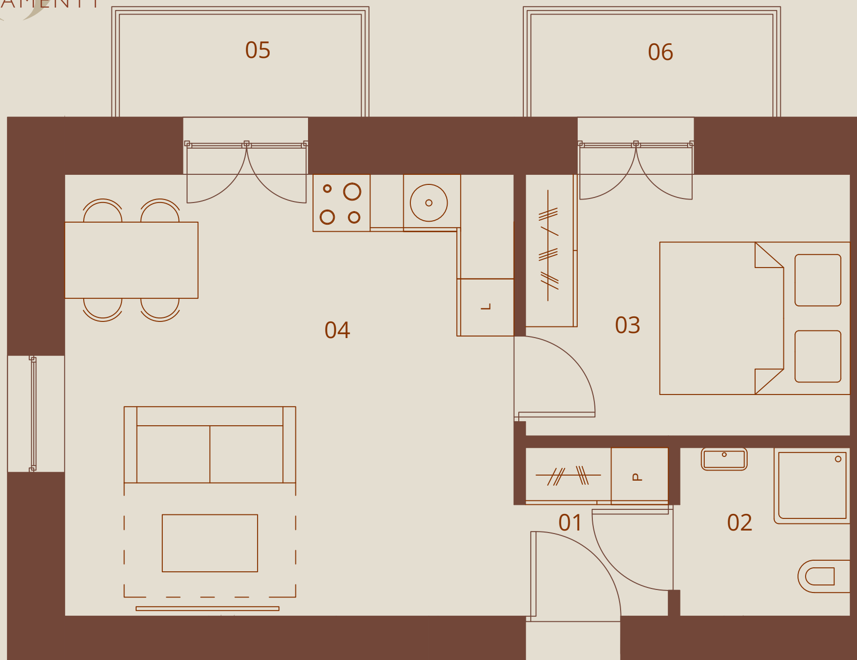
Plan piętra 2-ego
