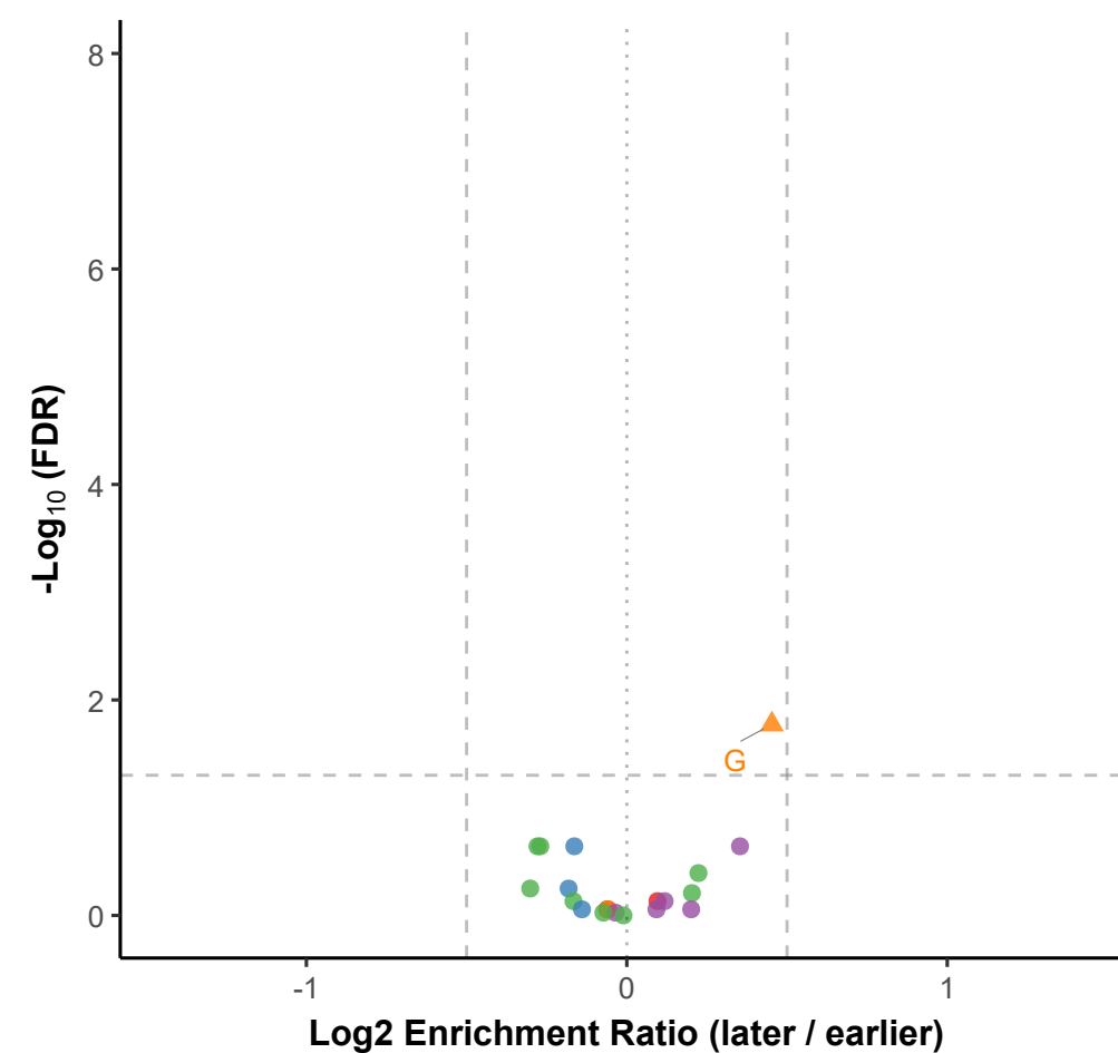
E-site | d10 vs d0
