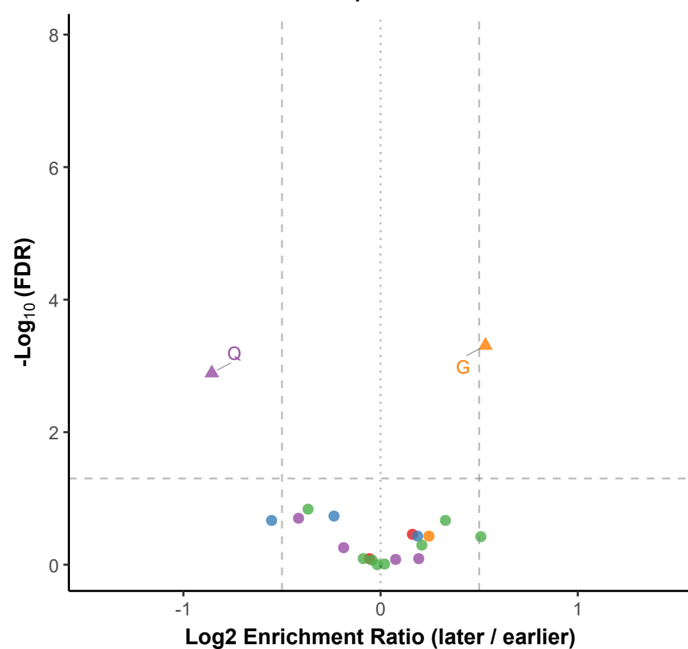
A-site | d10 vs d5
