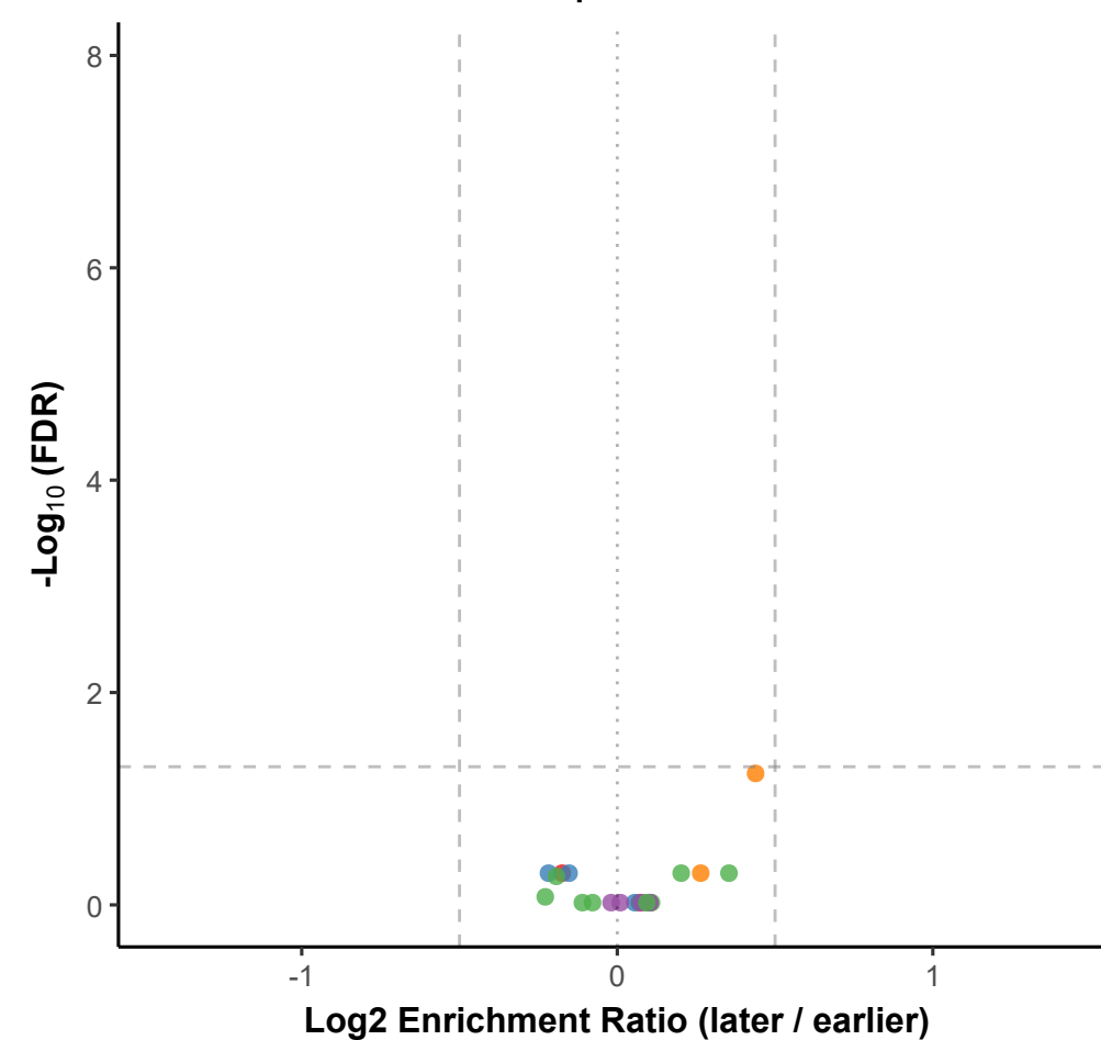
E-site | d10 vs d5
