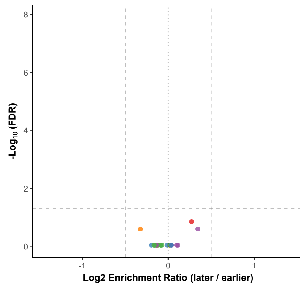
E-site | d5 vs d0
