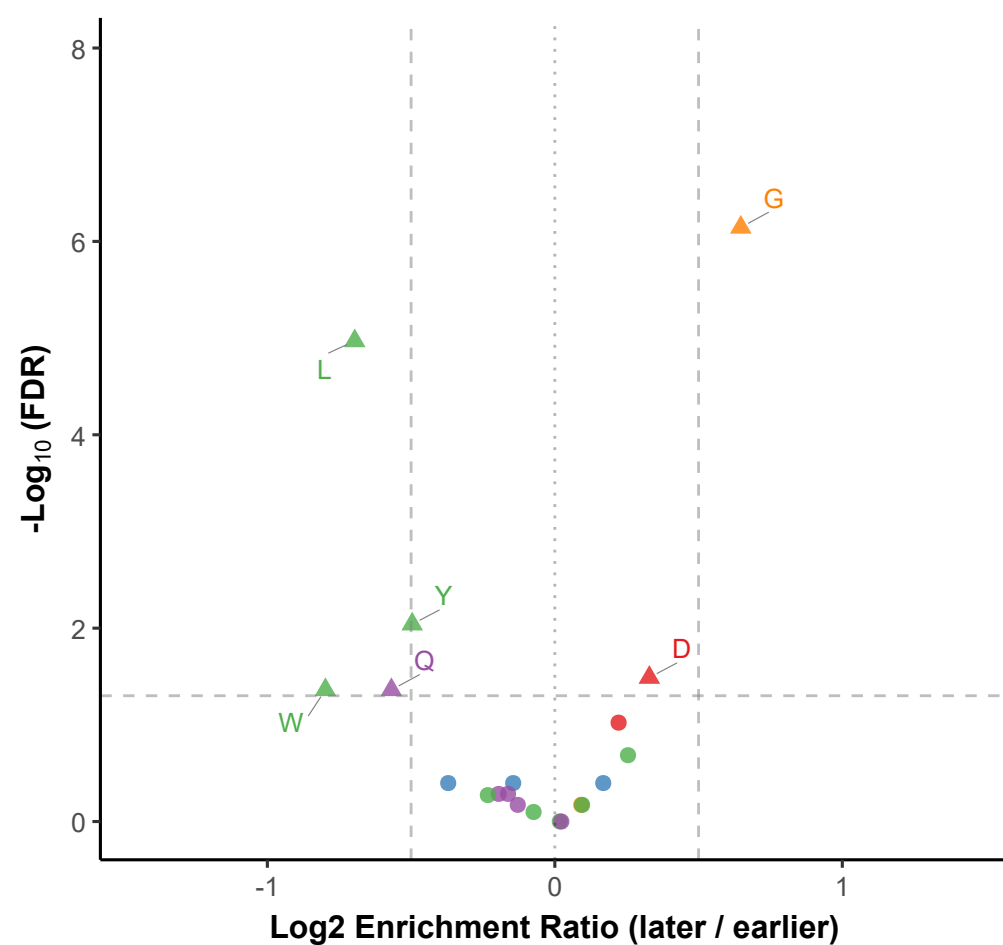
A-site | d10 vs d0
