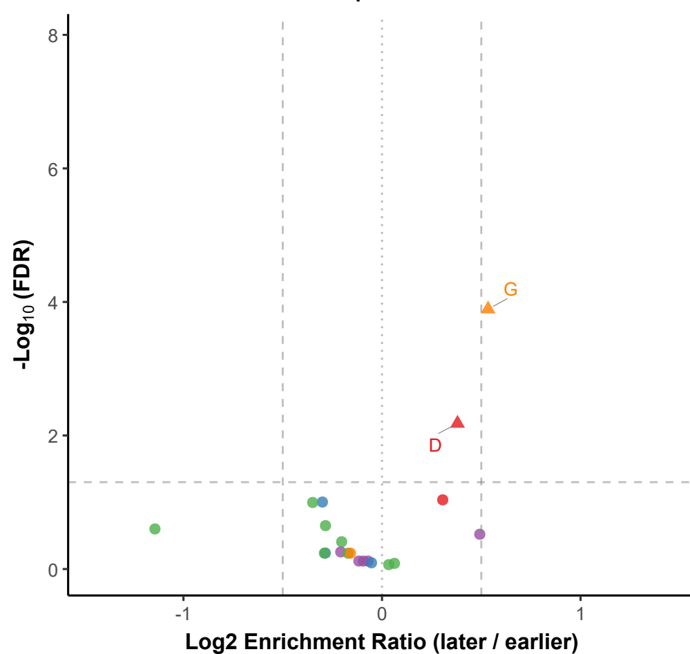
P-site | d10 vs d5
