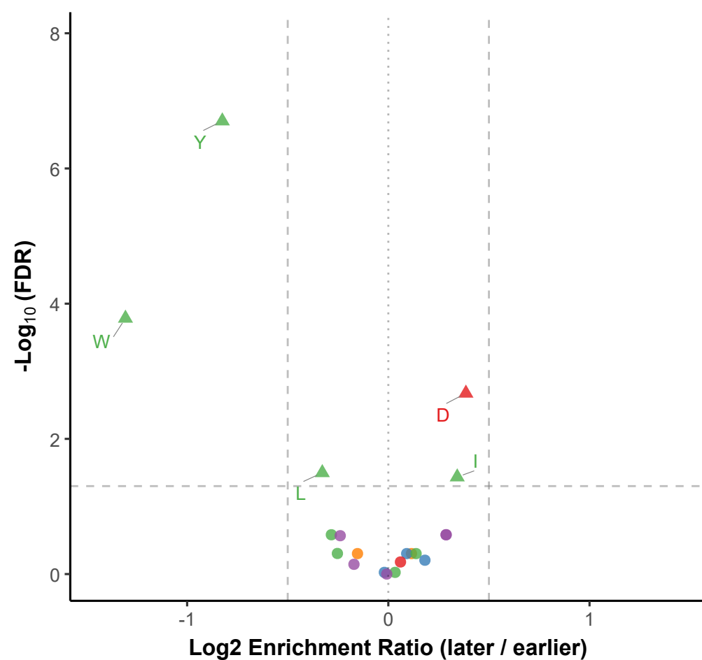
A-site | d5 vs d0
