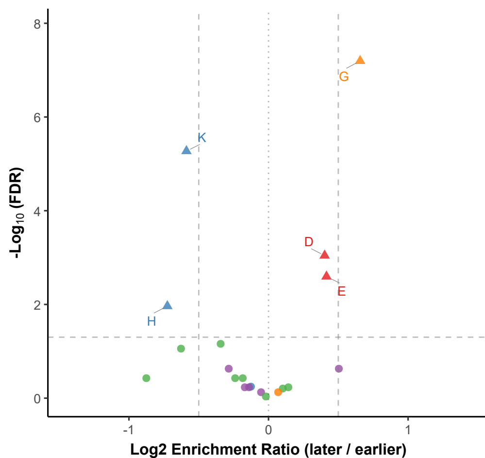
P-site | d10 vs d0
