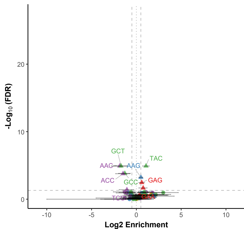
A-site | Day 0
