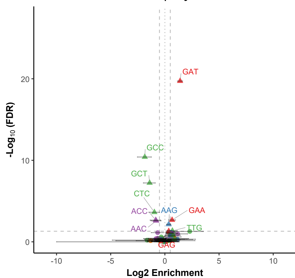
A-site | Day 5
