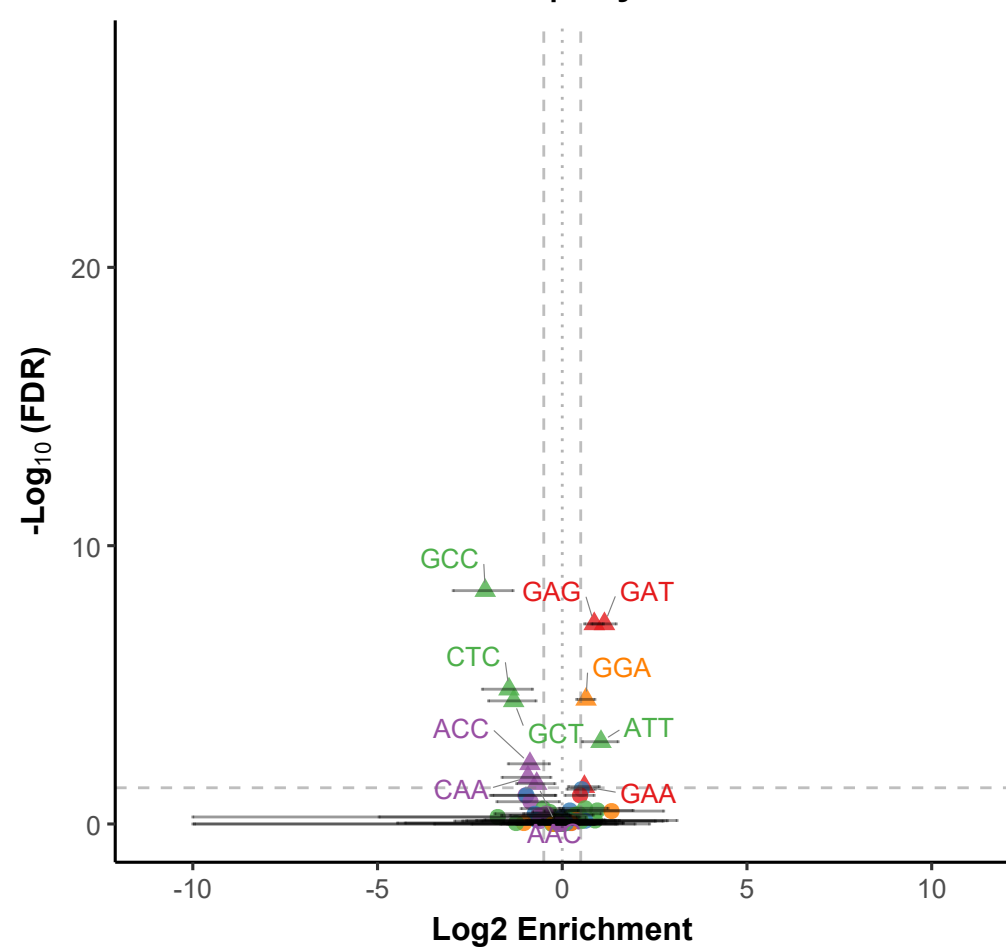
A-site | Day 10
