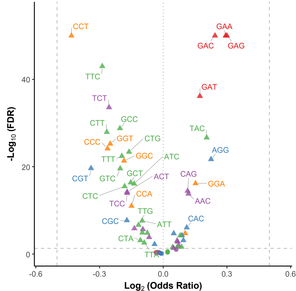
A-site
