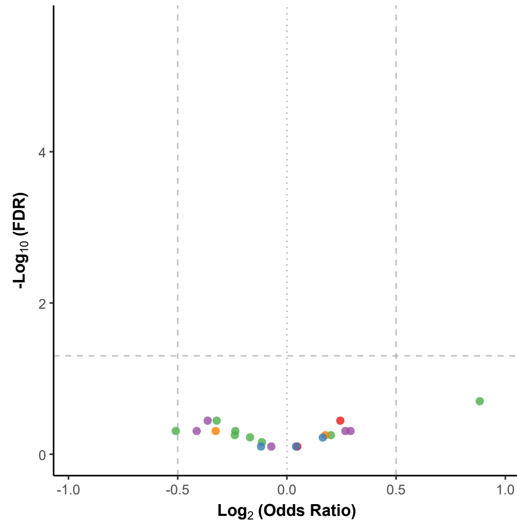
A-site
