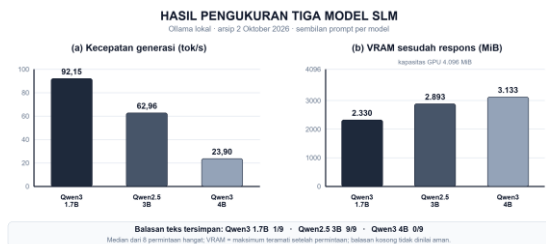
Gambar 3. (a) Median kecepatan generasi delapan permintaan hangat; (b) VRAM terbesar yang tercatat setelah permintaan. Jumlah balasan teks terlihat ditampilkan sebagai kontrol kualitas data [14].
