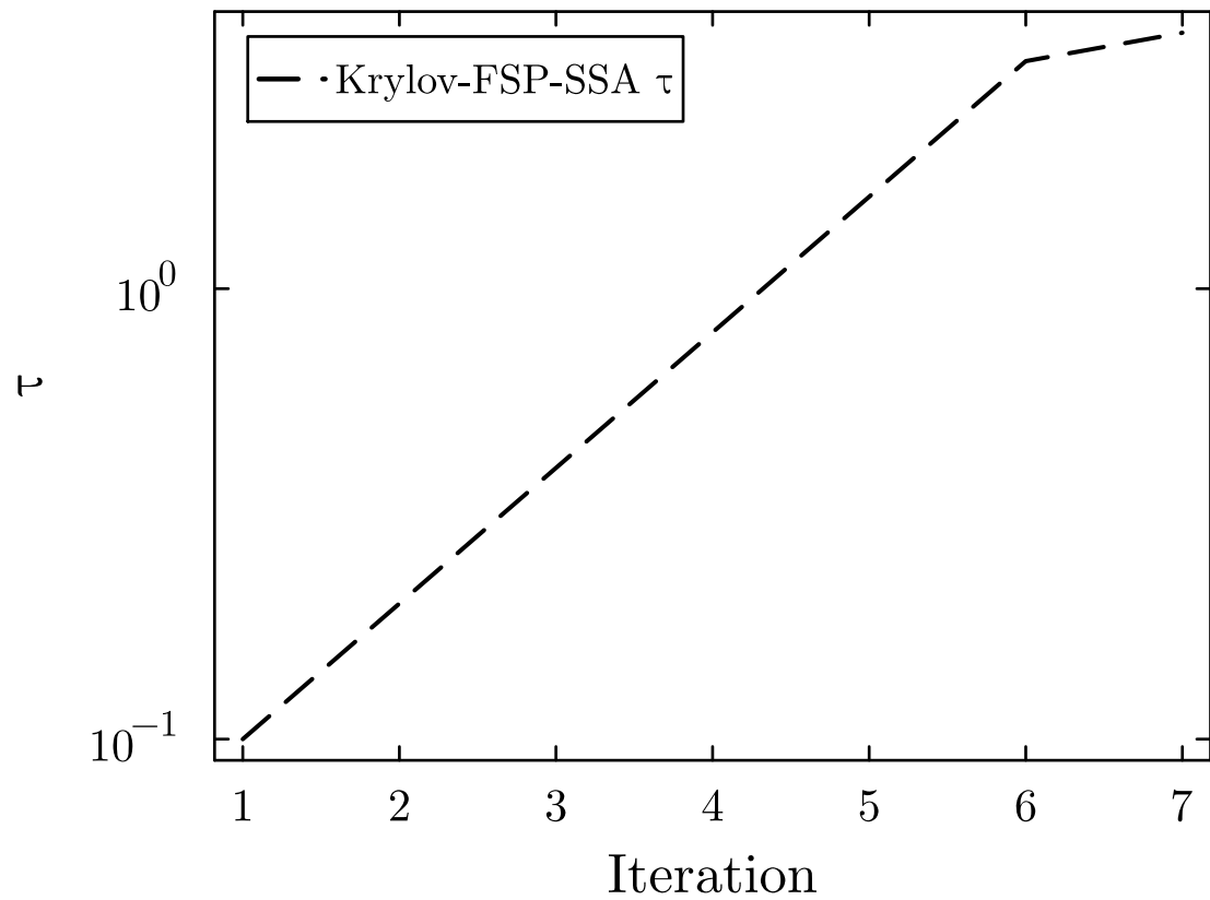
(b) Krylov-FSP-SSA time step
