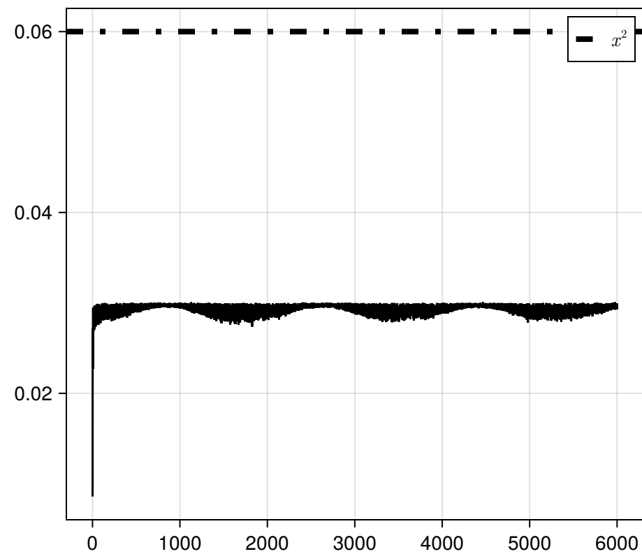
Lotka Volterra
