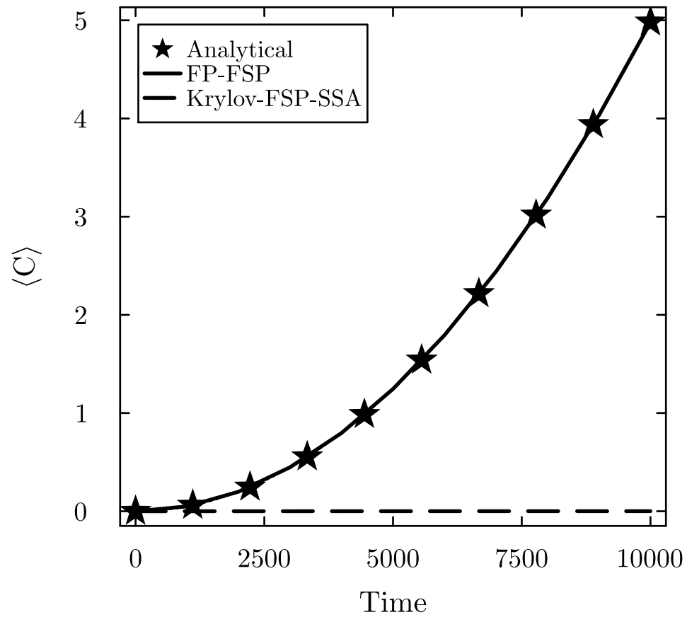
(b) Bottleneck
