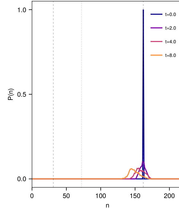
Multigrid FSP: P(n) at voxel 2 (hi→?)
