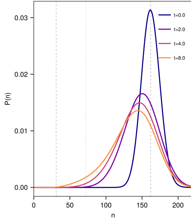
Per-voxel FSP: P(n) at voxel 2 (hi→?)
