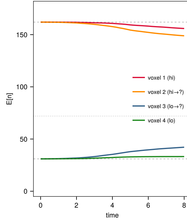
3. Multigrid FSP (V-cycle) (joint P(n_1, n_2) : correct front diffusion)
