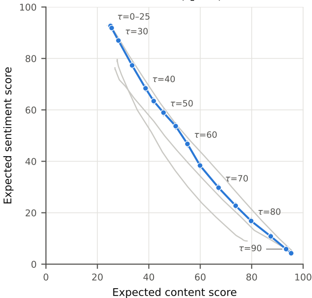
R-REBEL ( \ell_1 -std)
