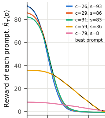
R-REBEL ( \ell_1 -std)
