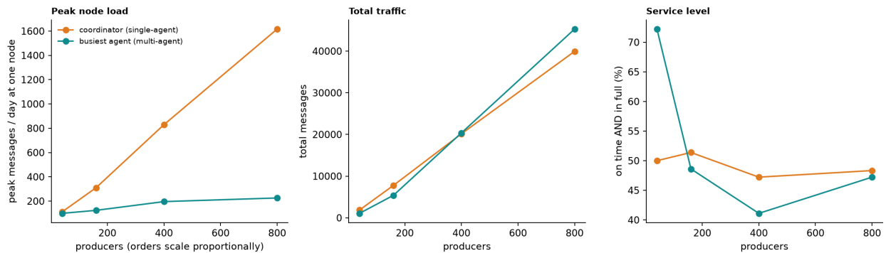
Gambar 10. Skala (Xpora): beban puncak per node, total pesan, dan OTIF ketika produsen dan order bertambah (fan-out CFP acak 25 produsen).
