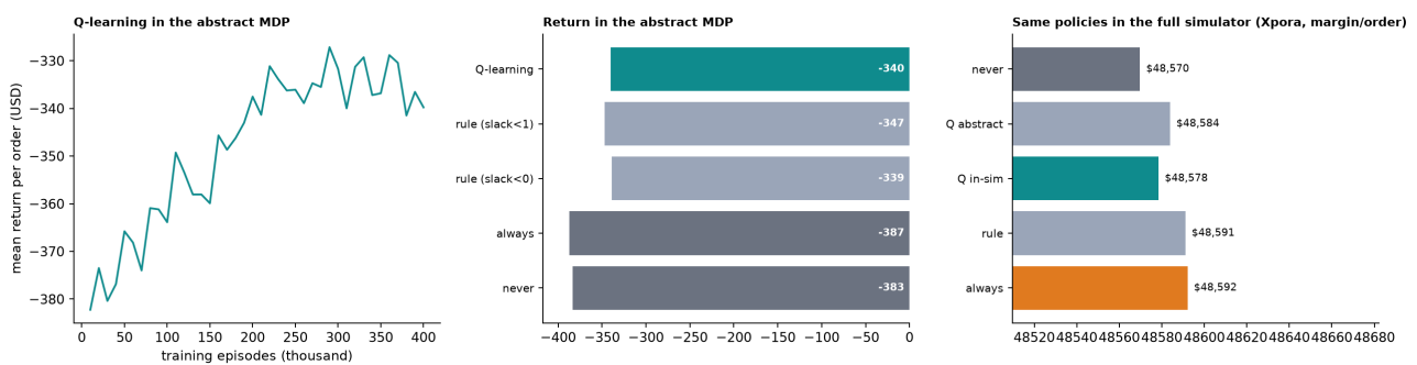
Gambar 17. Q-learning: kurva belajar di MDP abstrak, perbandingan policy di MDP, dan perbandingan policy yang sama di simulator penuh (Xpora).
