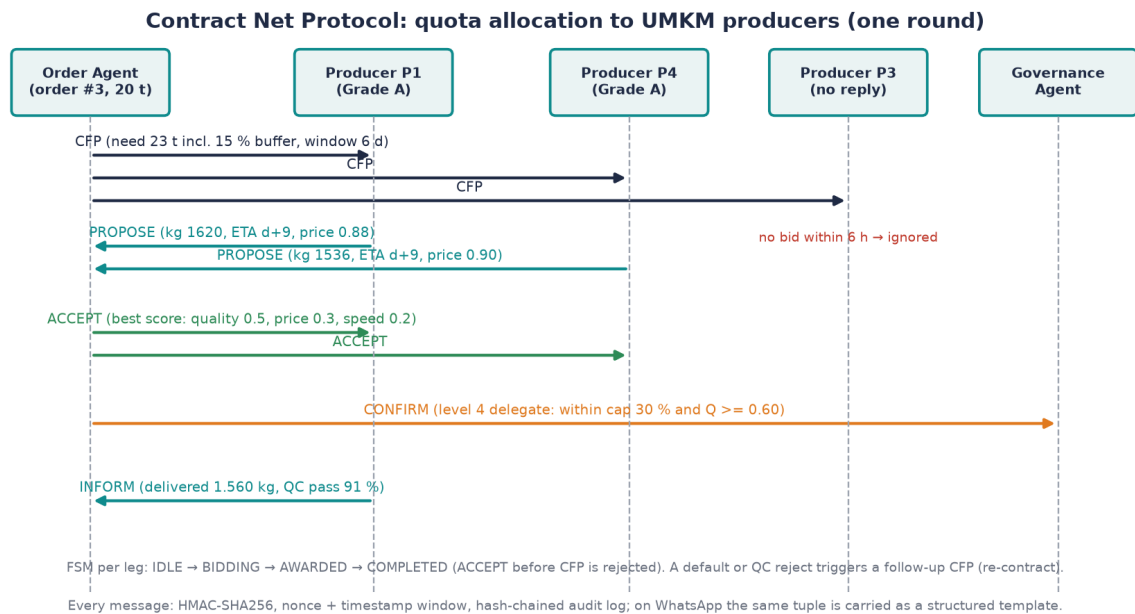
Gambar 4. Contract Net Protocol untuk kuota produsen UMKM; tiap leg divalidasi FSM dan ditandatangani HMAC.
