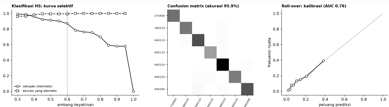
Gambar 16. Klasifikasi HS (kurva selektif dan confusion matrix) dan kalibrasi model roll-over.
