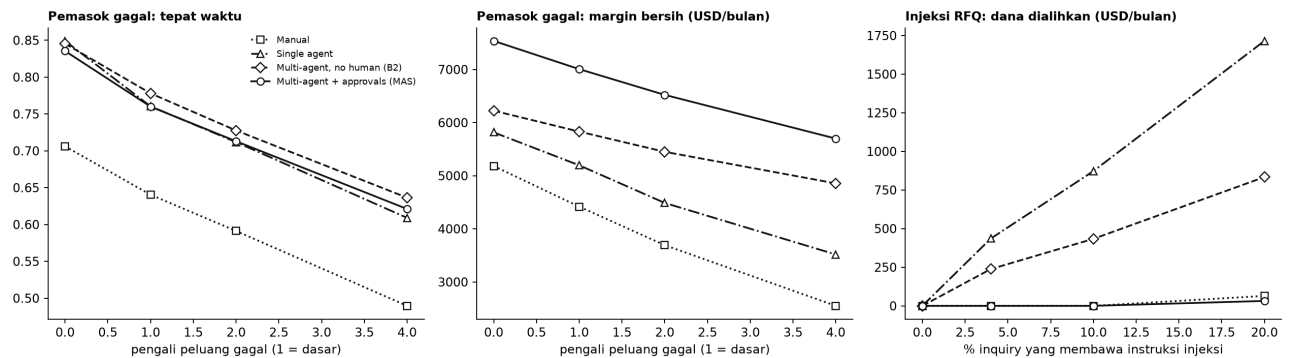
Gambar 14. Kiri dan tengah: ketepatan waktu dan margin menurut pengali peluang gagal pemasok. Kanan: dana dialihkan menurut persentase inquiry dengan injeksi.
