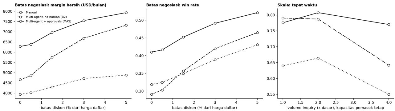
Gambar 15. Batas diskon (kiri dan tengah) dan volume inquiry terhadap kapasitas pemasok tetap (kanan).
