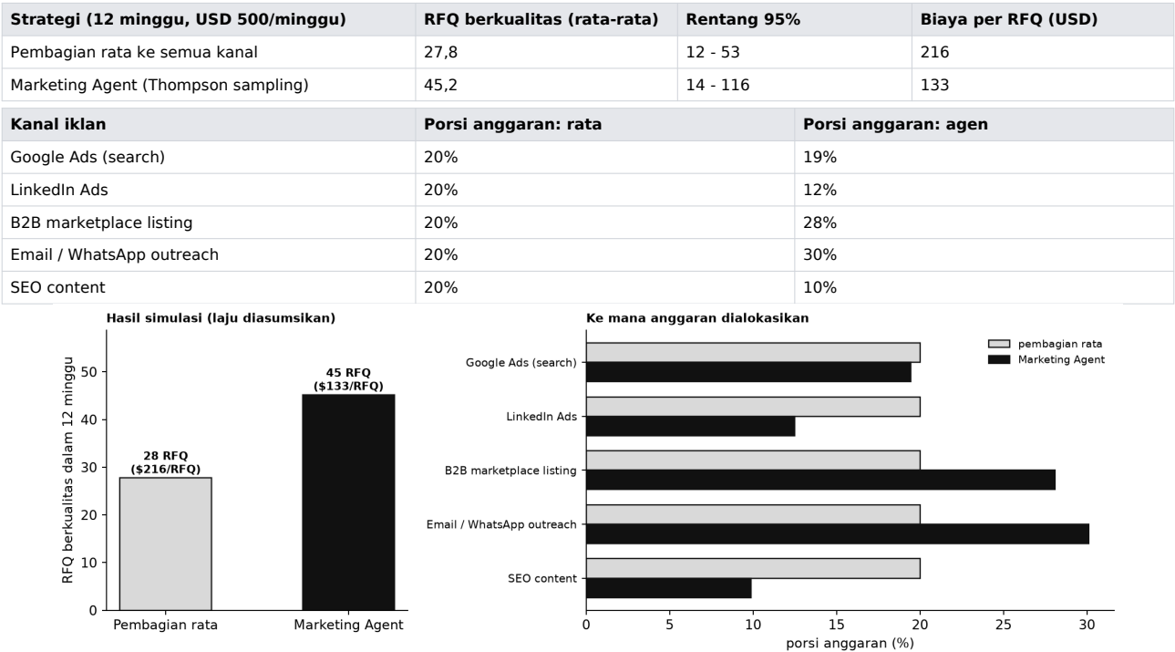
Gambar 17. Marketing Agent: RFQ berkualitas selama 12 minggu dan pembagian anggaran per kanal (400 pengulangan).
