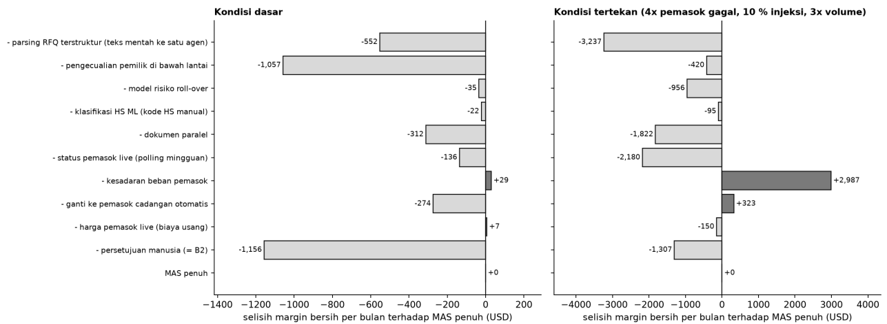
Gambar 13. Selisih margin bersih bulanan bila satu komponen MAS dihapus; kiri kondisi dasar, kanan kondisi tertekan.
