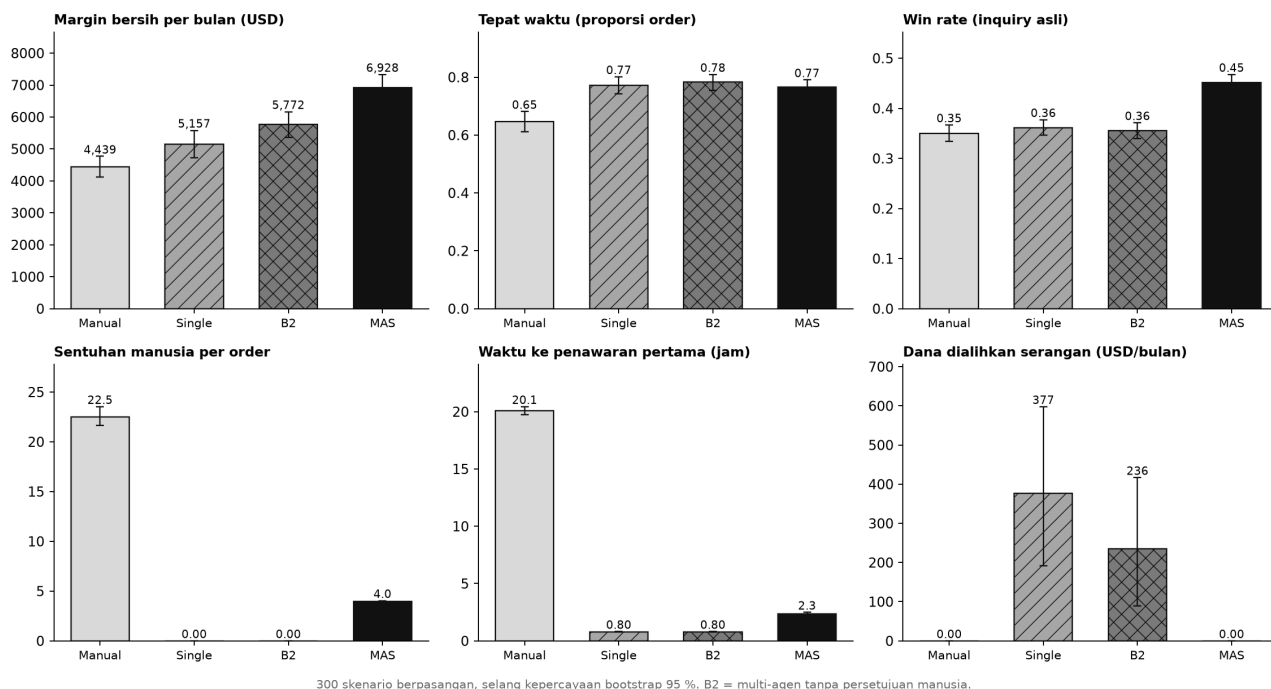
Gambar 12. Hasil utama pada 300 skenario berpasangan, dengan selang kepercayaan 95%.
