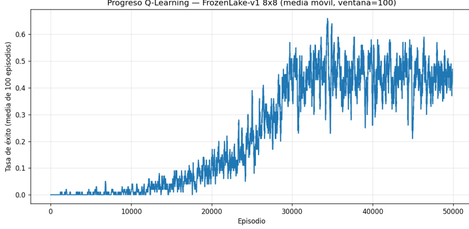
Figure 1: Fase 1: media móvil (ventana 100) de la recompensa por episodio en FrozenLake-v1 8 \times 8 resbaladiza. El aprendizaje despegue hacia el episodio \sim 20k y se estabiliza en torno a 0.45–0.50.
