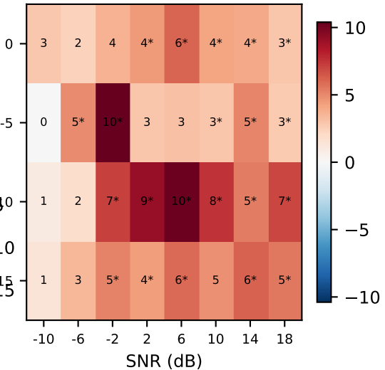
A5 – A0 (pp)
