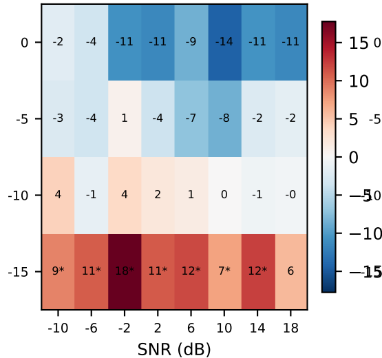
A5 – MCLDNN (pp)
