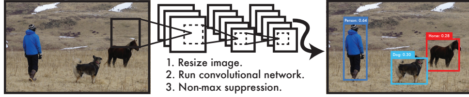
FIGURE 11 – Principe de détection de YOLO : traitement en un seul passage ( Single-Shot ) sur une grille spatiale. Extrait de Redmon et al. (2016).
