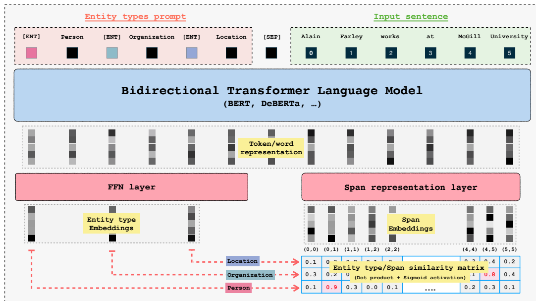
FIGURE 15 – Architecture globale du modèle GLiNER : comparaison entre les morceaux de texte et les entités recherchées. Extrait de Zaratiana et al. (2024). Ce schéma est également disponible en grand format horizontal en Annexe D.
