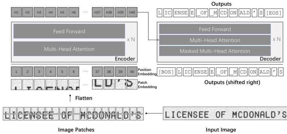
FIGURE 10 – Architecture hybride de TrOCR : l'image de la ligne (imprimée ou manuscrite) est découpée en patches visuels traités par un encodeur Transformer, puis transcrite par un décodeur de texte. Extrait de Li et al. (2023).
