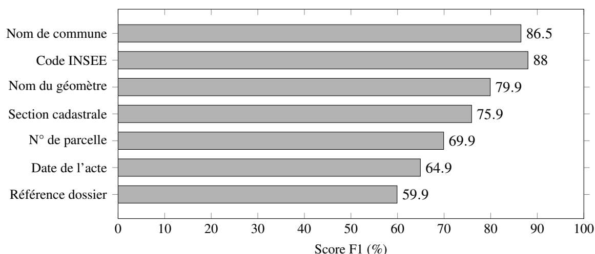
FIGURE 39 – Scores F1 par champ d'indexation, mesurés sur le jeu de test de 33 documents. La commune et le code INSEE bénéficient du filtrage par distance de Levenshtein contre le référentiel INSEE. La date et la référence de dossier (rarement sur le document) sont les champs les moins bien lus, notamment sur les actes manuscrits.
