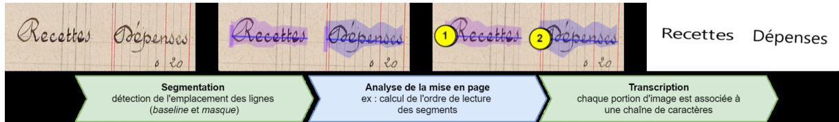
FIGURE 8 – Étapes de traitement d'un système HTR : segmentation de la page en lignes, analyse de la mise en page, puis transcription de chaque portion d'image en texte. Extrait de Chagué et al. (2021).
