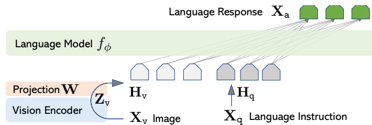
FIGURE 18 – Architecture interne du modèle Vision-Language LLaVA. Extrait de Liu et al. (2024). Une version grand format est disponible en Annexe E.
