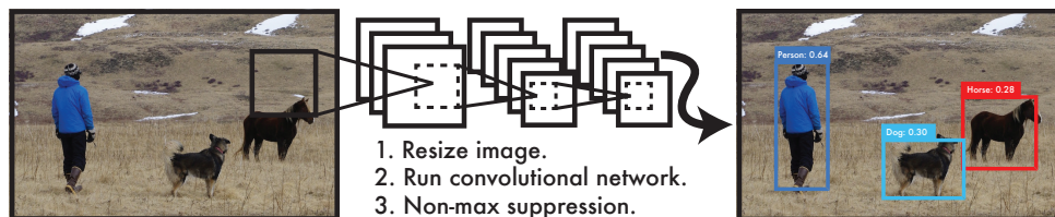
FIGURE 11 – Principe de détection de YOLO : traitement en un seul passage sur une grille spatiale. Extrait de Redmon et al. (2016).
