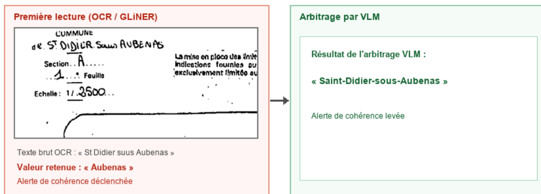
FIGURE 25 – Arbitrage par le modèle VLM déclenché par une alerte de cohérence sur le document du Géomètre B (EXEMPLE_GEOMETRE_B.pdf).
