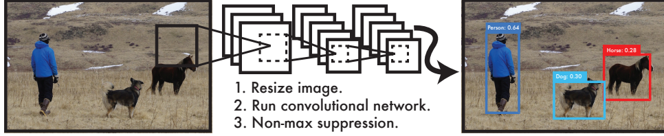
FIGURE 11 – Principe de détection de YOLO : traitement en un seul passage ( Single-Shot ) sur une grille spatiale. Extrait de Redmon et al. (2016).
