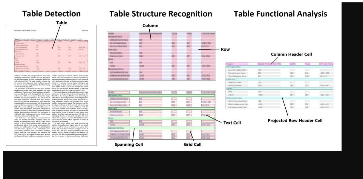
FIGURE 19 – Les trois tâches du Table Transformer de Smock et al. (2022) : détection de la table dans la page (gauche), reconnaissance de sa structure en lignes et colonnes (centre), et analyse fonctionnelle des types de cellules (droite). Source : dépôt officiel Microsoft Table Transformer.
