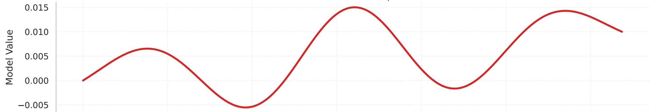
True Model: \delta v_s(r)
