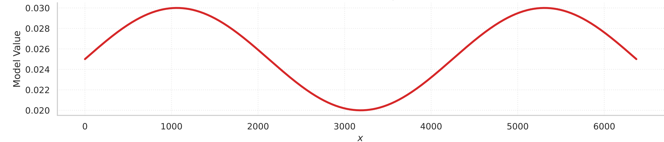
True Model: \delta \rho(r)
