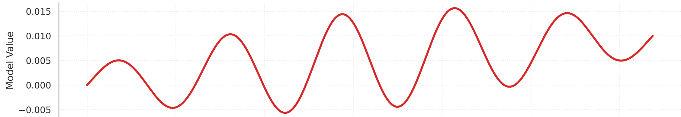
True Model: \delta \rho(r)
