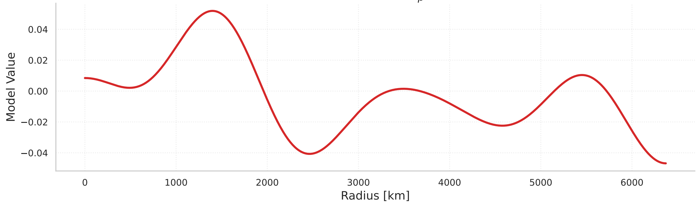
True Model: \delta v_p(r)
